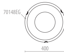
70148 Ø 400 - VE/PU: 1 2 x 60 W - E27 - 230V
