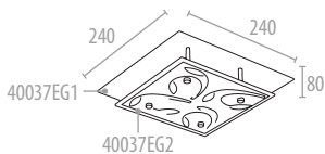
40037 240 x 240 x 80 - VE/PU: 5 1 x 60 W - E27 - 230V
