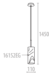
16152-1 Ø 110, ↓ 1450 - VE/PU: 18 1 x 60 W - E27 - 230V
