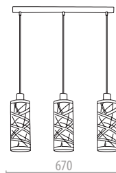
16166-3 ↔ 670 - VE/PU: 3 3 x 60 W - E27 - 230V
