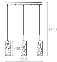
16152-3 ↔ 650, ↓ 1450 - VE/PU: 3 3 x 60 W - E27 - 230V
