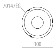
70147 Ø 300 - VE/PU: 1 1 x 60 W - E27 - 230V
