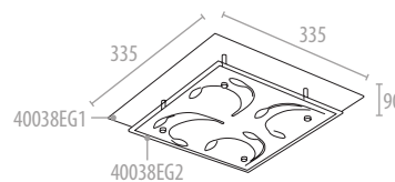
40038 335 x 335 x 90 - VE/PU: 4 2 x 60 W - E27 - 230V
