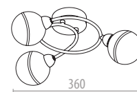
60750-3 360 x 315 x 145 • VE/PU: 12 3 x 33 W • G9 • 230V
