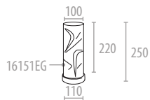
16151 Ø 110, ↑ 250 - VE/PU: 6 1 x 60 W - E27 - 230V
