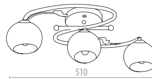
997106-3 510 x 350 • VE/PU: 4 3 x 60 W • E27 • 230V
